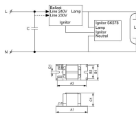
Caractéristiques Philips Ballast Imprégné BSN 400 K407-ITS 230/240V 50Hz BC3-166
