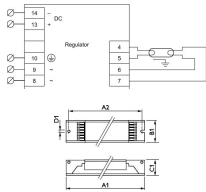
Technische Daten Philips HF-R 158 TL-D EII 220-240V für 1x58W
